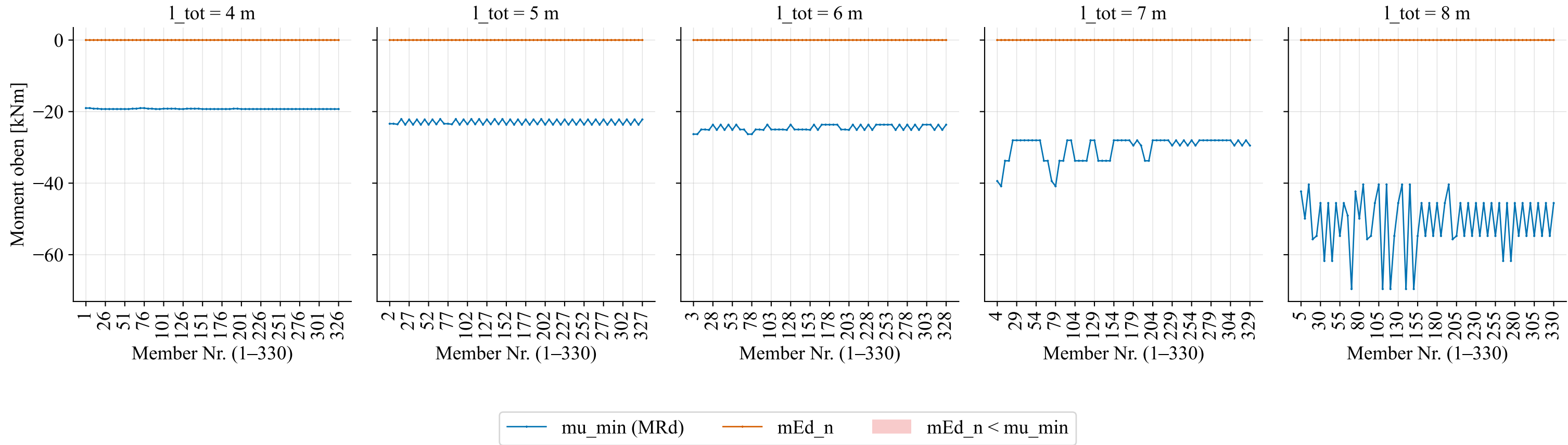
Biege widerstand \mu_{\min} (MRd) vs. Bemessungsmoment mEd_n je Member, kategorisiert nach Spannweite (Members_rc_rec_simple_massiv)
